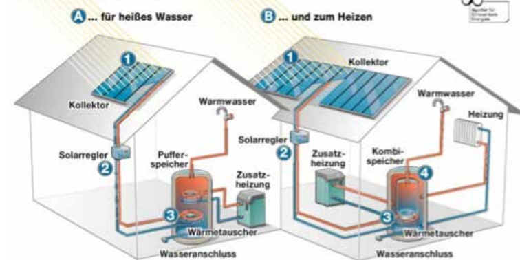
A Solaranlag fir d'Produktioun vu waarmem Waasser
